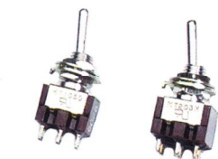
MM518 MM520 Mighty Mite® Mini Toggles 518(SPDT) (520DPDT)
